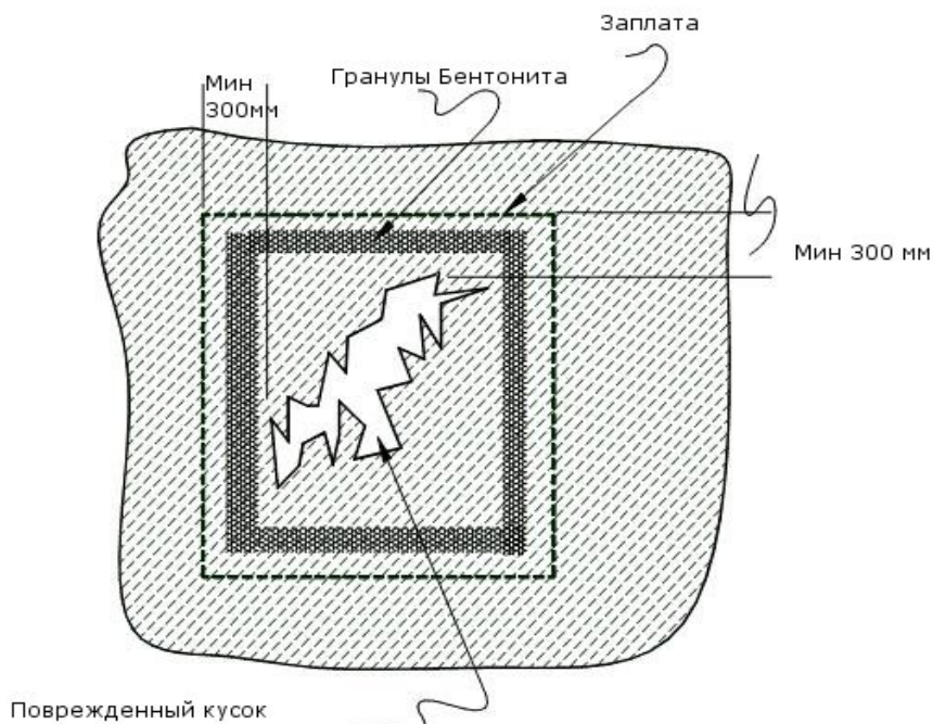
Рисунок 5. Устранение повреждений
